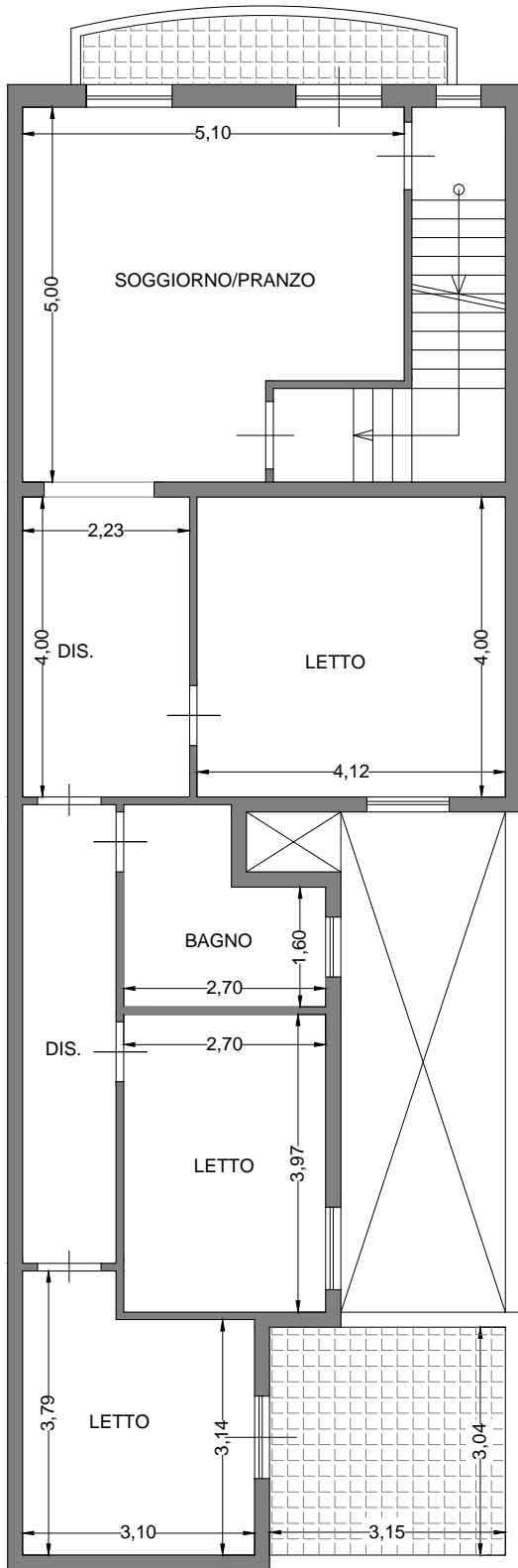
PIANTA APPARTAMENTO VIA DONIZETTI 15 PIANO 1° - 2° SCALA 1:100
