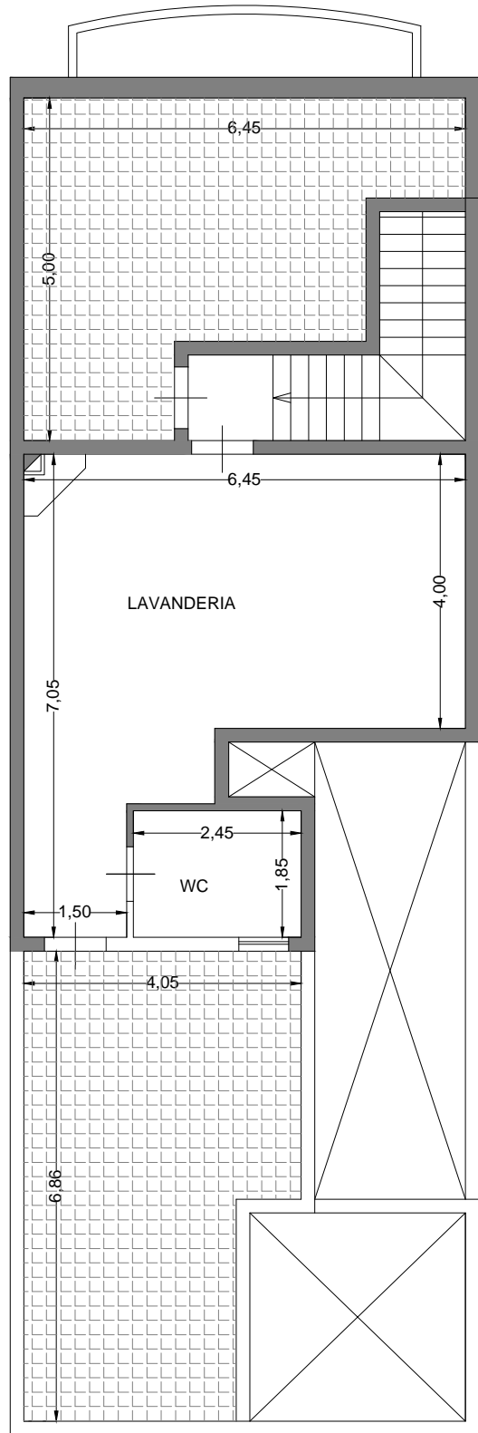
PIANTA APPARTAMENTO VIA DONIZETTI 15 PIANO 1° - 2° SCALA 1:100
