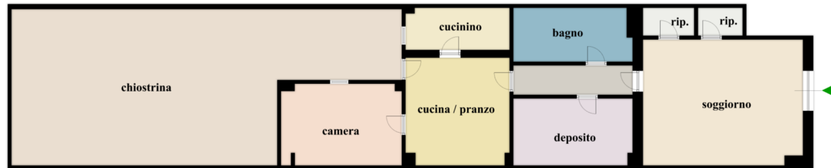
PIANO TERRA CON MODESTE MODIFICHE INTERNE
